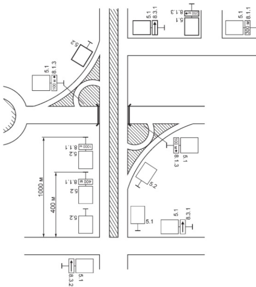
Рисунок В.5 — Пример расстановки знаков 5.1 и 5.2
