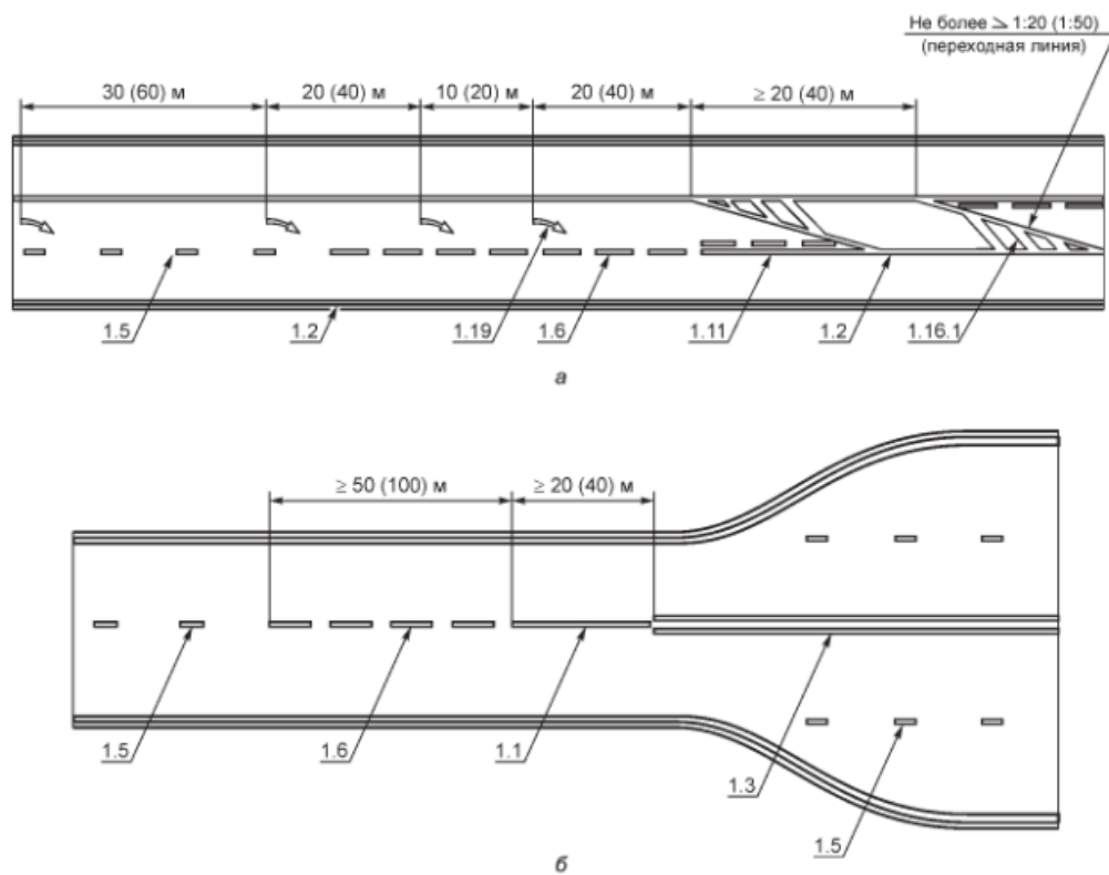
Рисунок В.8 — Пример нанесения разметки при уменьшении и увеличении количества полос для движения в одном направлении
