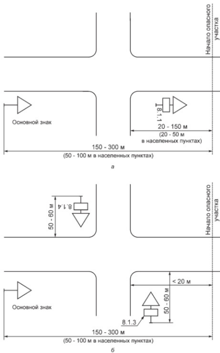
Рисунок В.2 — Установка предупреждающих знаков
