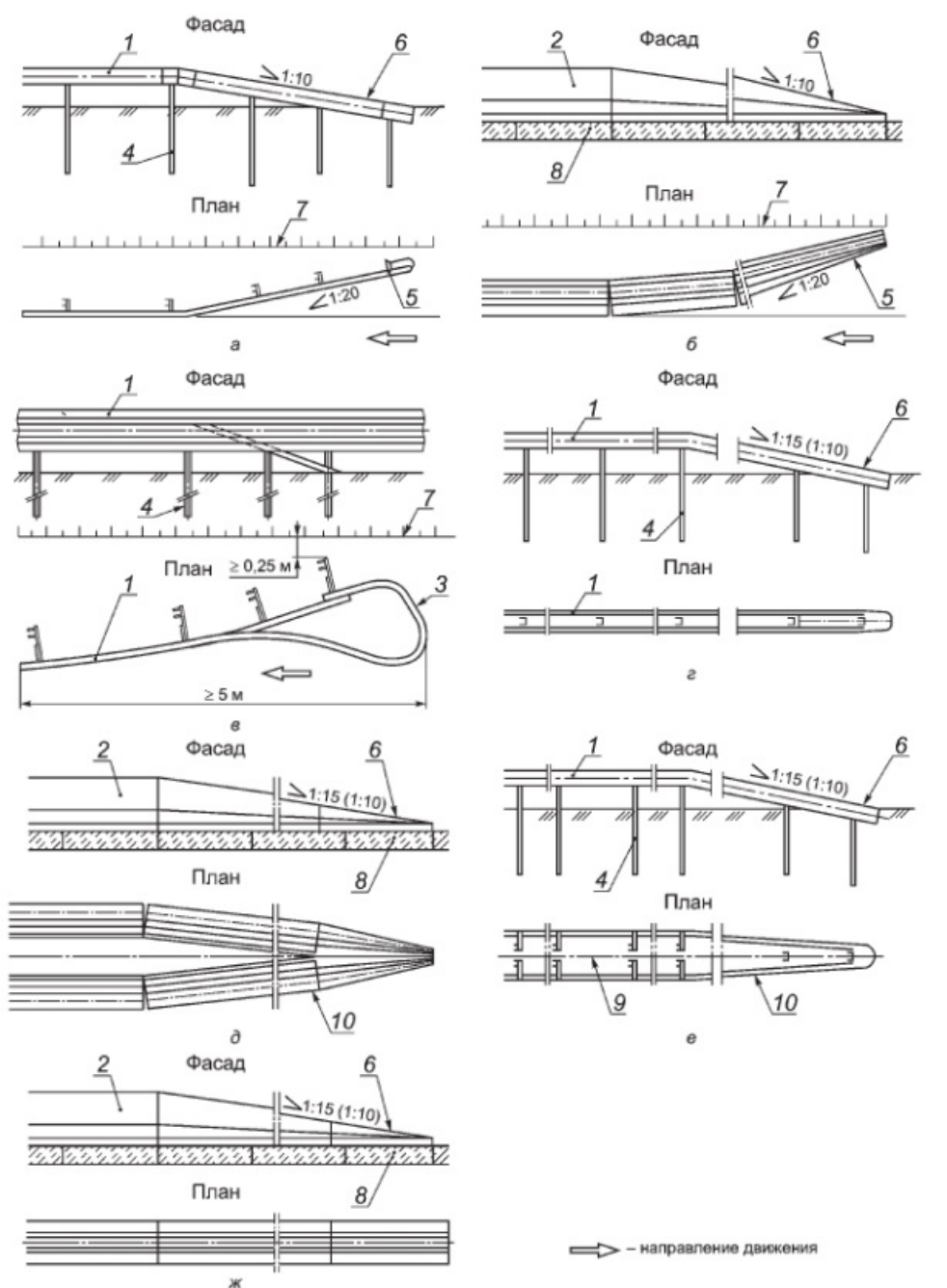
1 — барьерное ограждение; 2 — паралетное ограждение; 3 — изгиб балки ограждения; 4 — стойка ограждения; 5 — отгон ограждения; 6 — понижение ограждения на начальном и конечном участках; 7 — бровка земляного попутна; 8 — основание; 9 — ось разделительной полосы; 10 — сближение рядов ограждения с осью разделительной полосы
