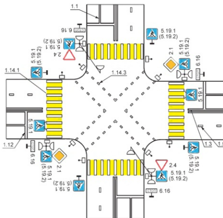
Рисунок В.19 — Пример нанесения диагонального пешеходного перехода
