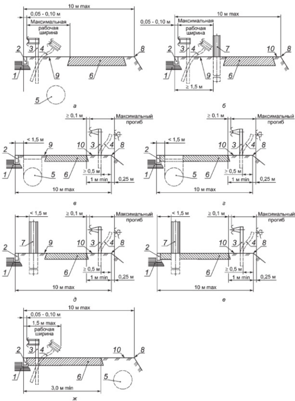
1 — проезжая часть; 2 — бордюрный камень; 3 — недеформированное ограждение; 4 — деформированное ограждение; 5 — подземные инженерные сети; 6 — тротуар; 7 — массивная опора; 8 — бровка земляного полотна или край подпорной стены; 9 — газон; 10 — полоса между тротуаром и бровкой земляного полотна
