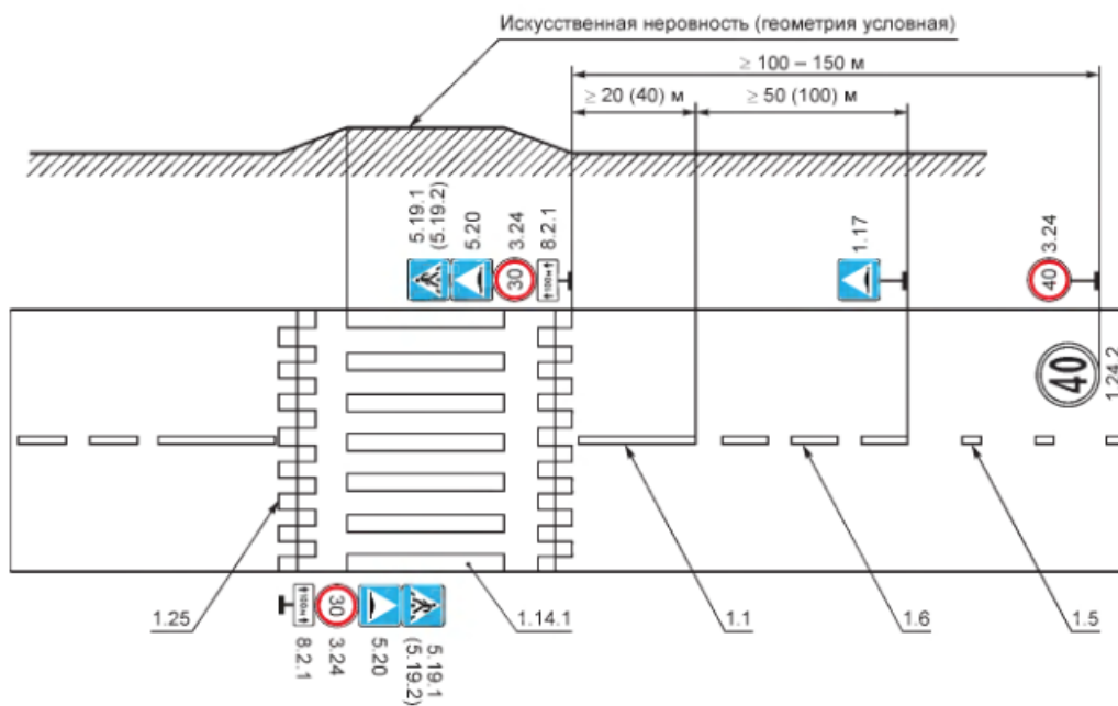
Рисунок В.21 — Пример нанесения разметки 1.25
