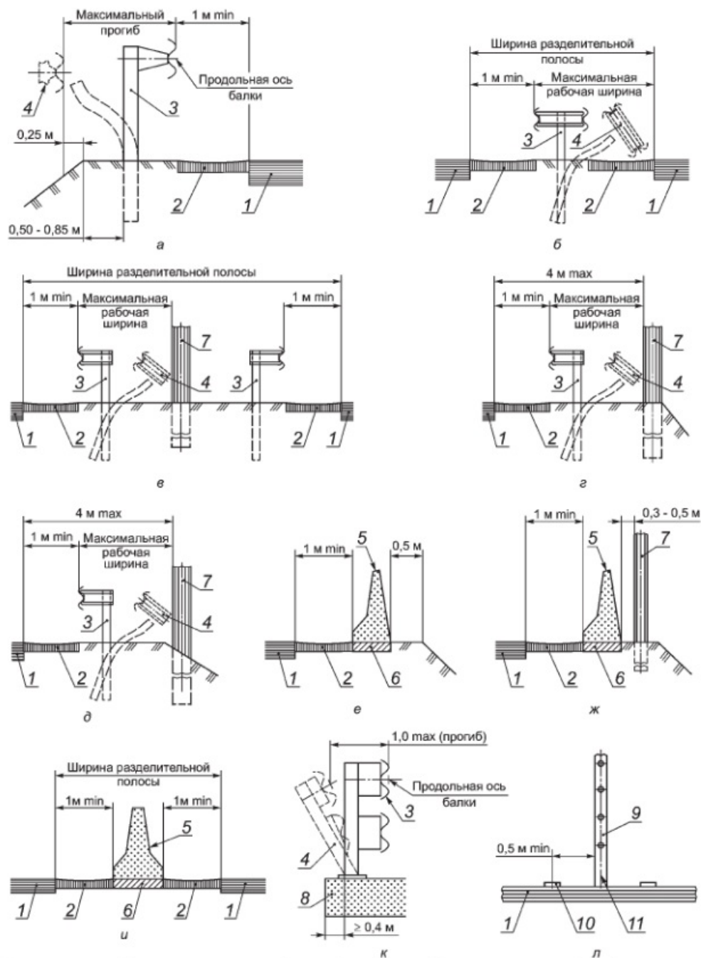
Рисунок В.28 — Примеры установки дорожных ограждений
