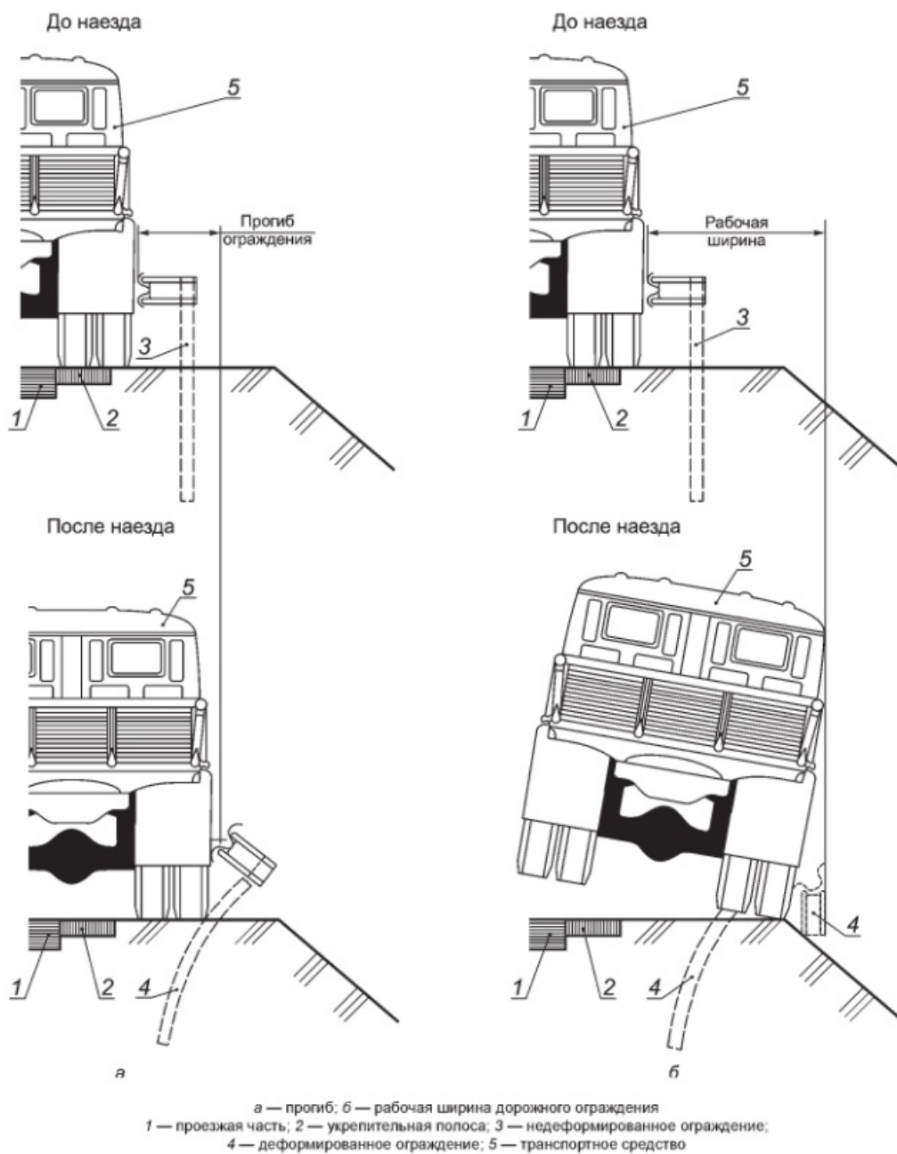
Рисунок В.27 — Смещение дорожного ограждения
