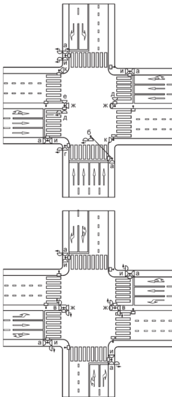
Рисунок В.26 — Места установки светофоров
