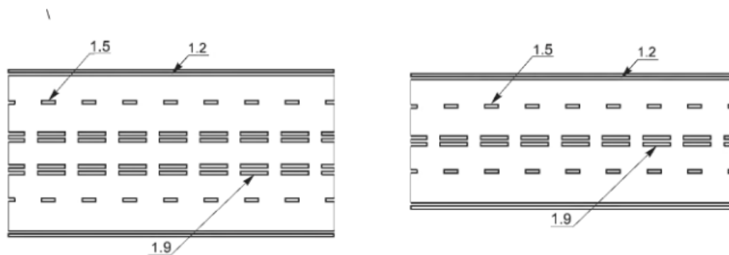
Рисунок В.17 — Примеры нанесения разметки 1.9
